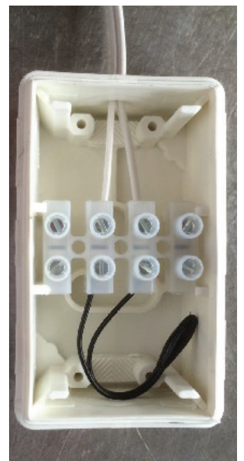
Uteføler og den hvite utefølerledningen samles med samlemuffen inne i samleboxen.
