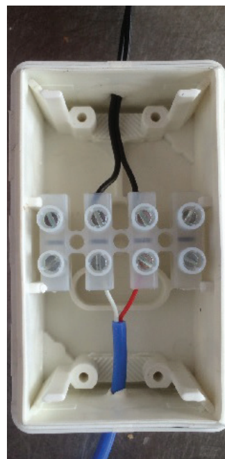
Solfangerføler og den svarte solfangeledning samles med samlemuffen inne i samleboxen.
